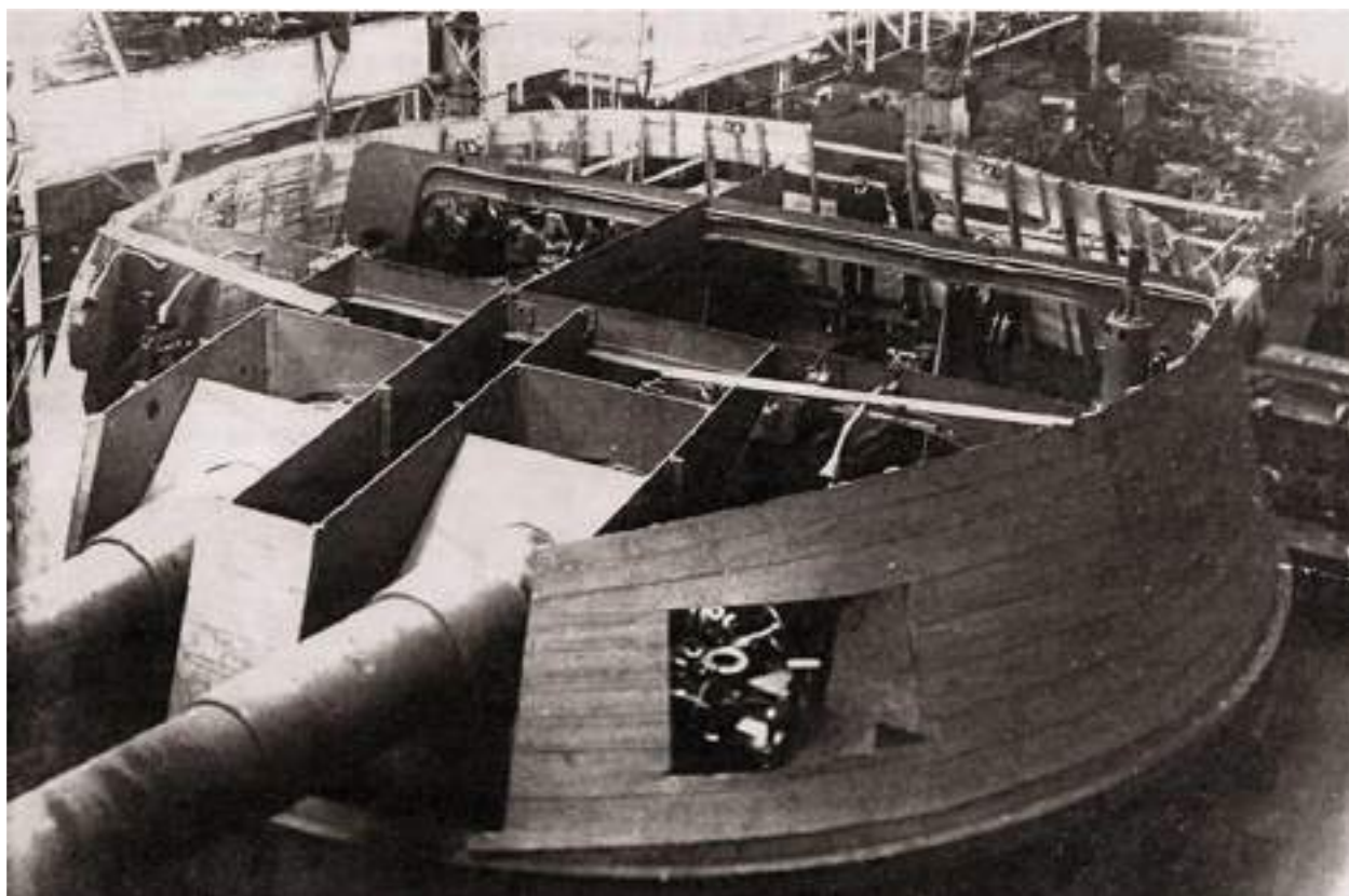
Строительство башни БМ-2-12.
